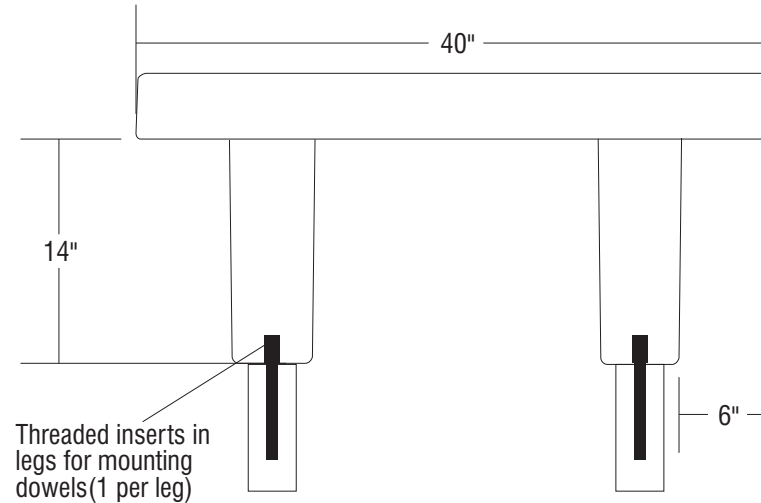
ELEVATION
