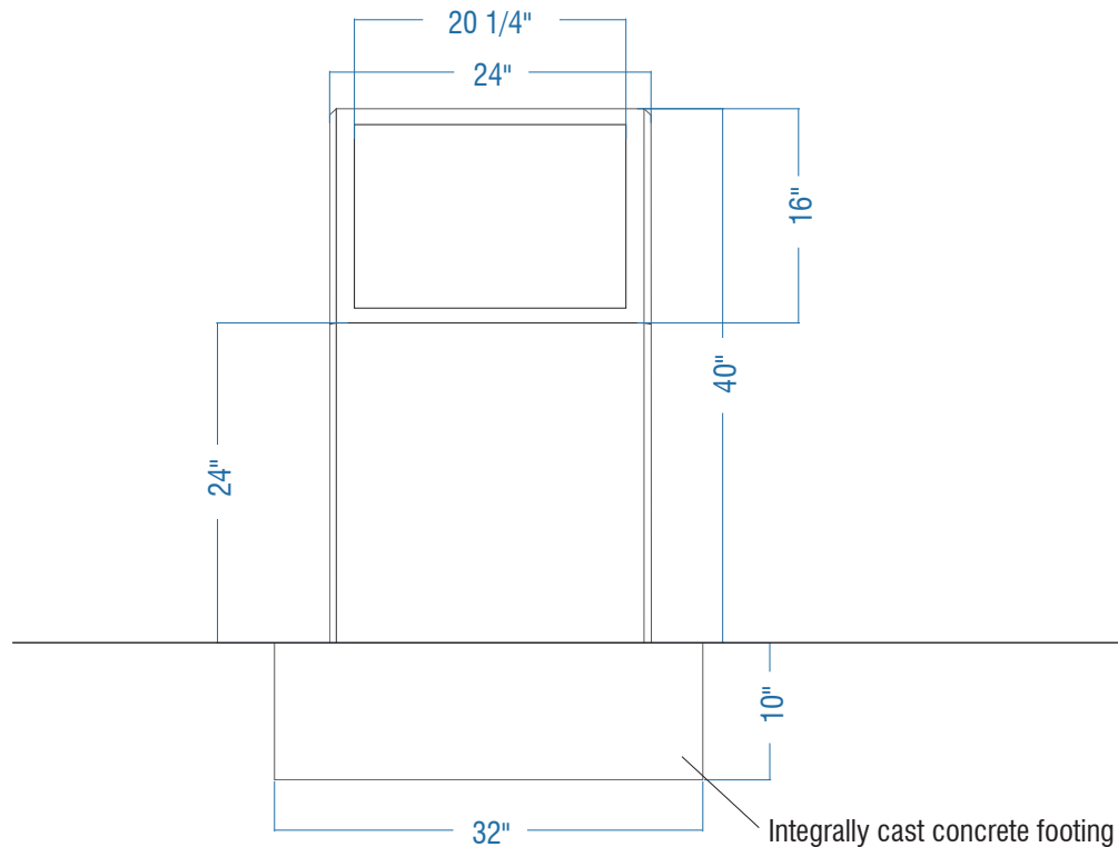
ELEVATION
